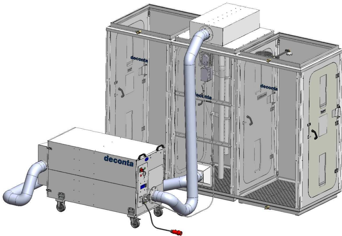
116088: 3 Kammer Schleuse Quick-Dush mit Luftdusche mit Luftregler
